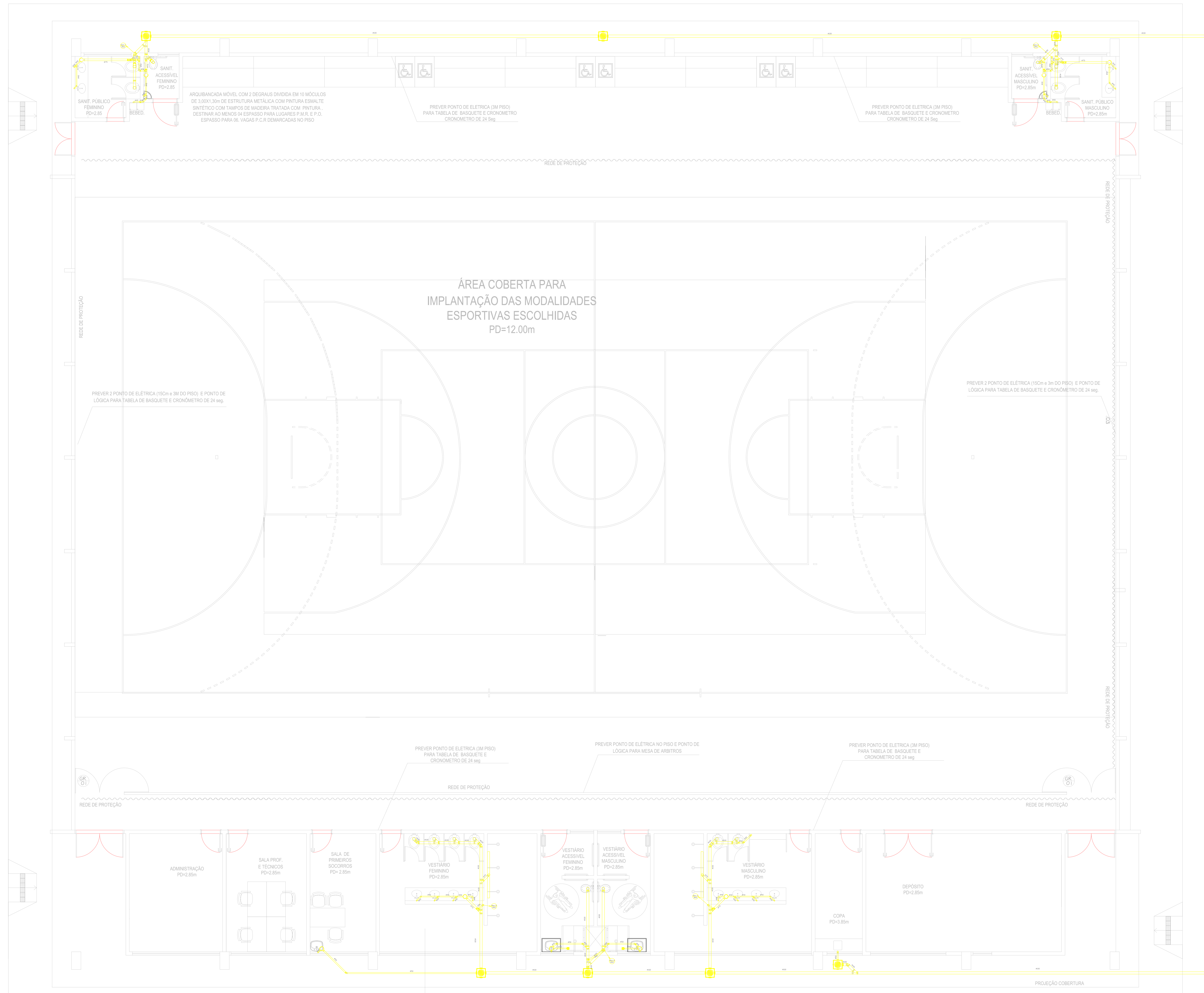
GINÁSIO PLANTA - PAV. TÉRREO ESC. 1:50
