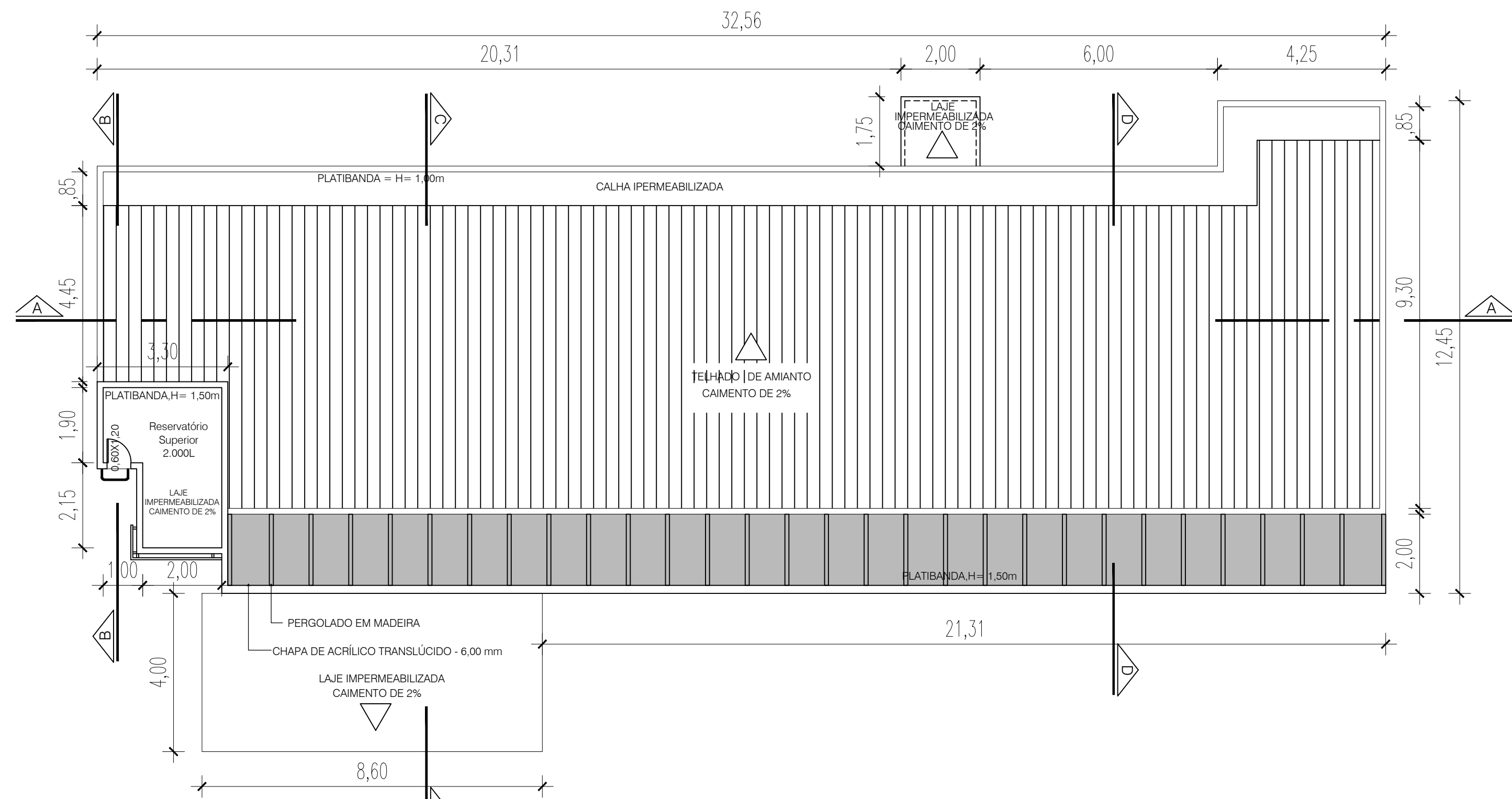
PLANTA DE COBERTURA ESCALA: 1/100
