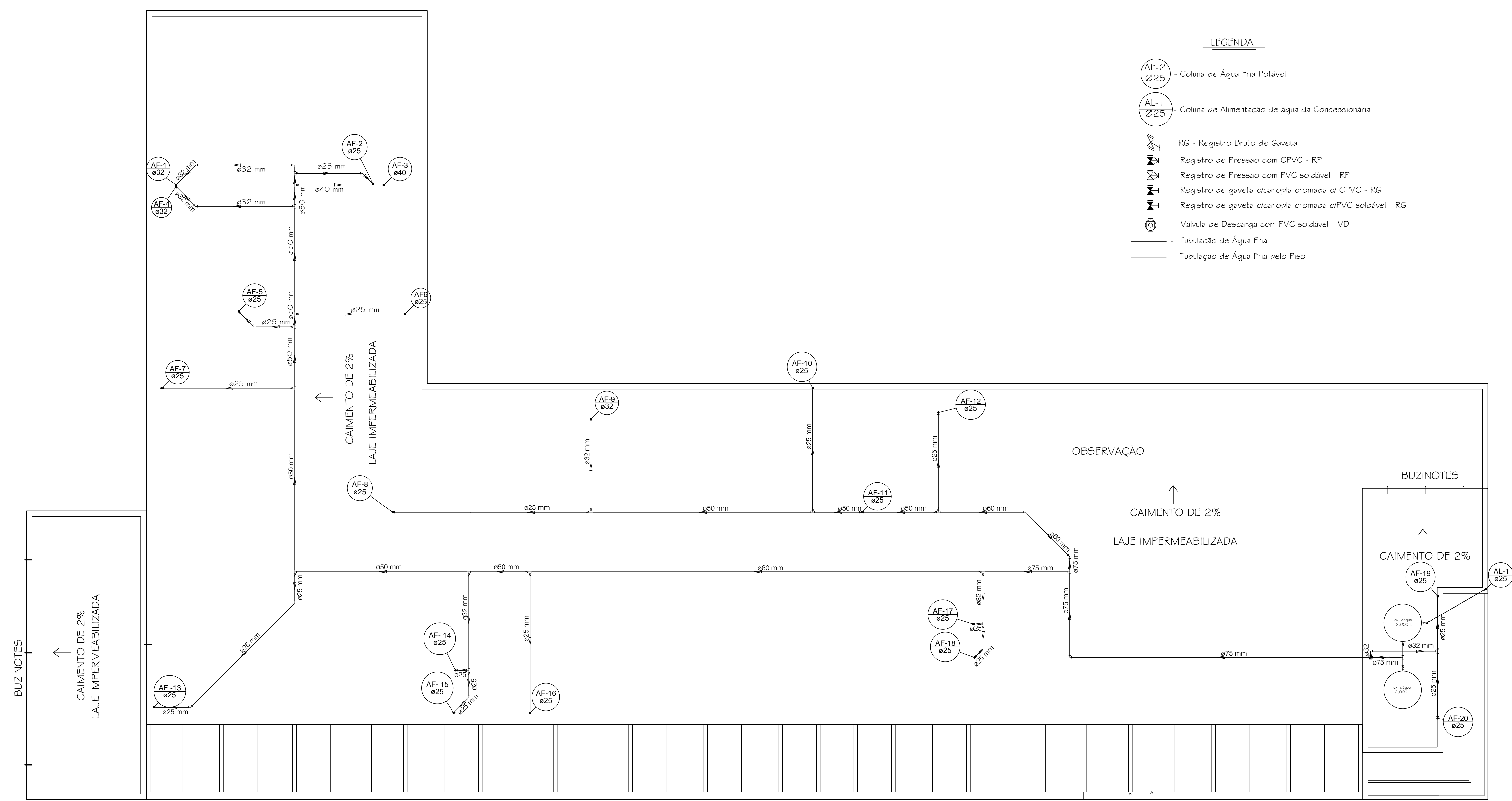
PLANTA DE COBERTURA ESC.: 1/50
