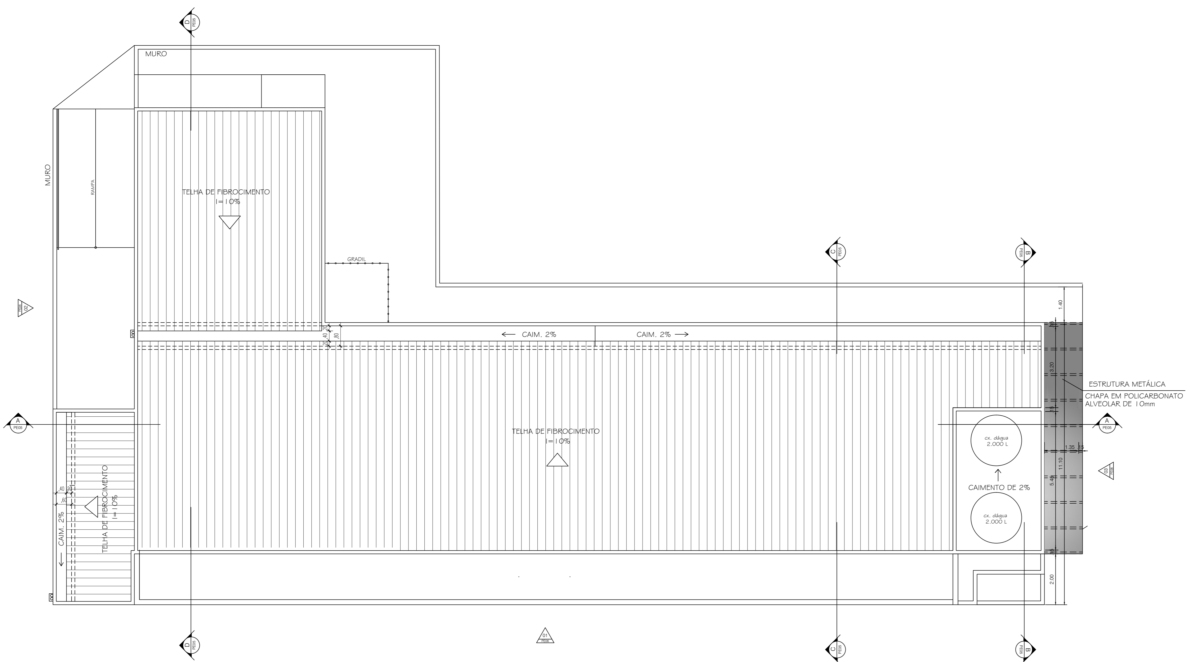
01 PLANTA BAIXA - COBERTURA PEB3 ESC. 1/75
